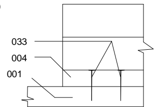
100 / 100 A-A
