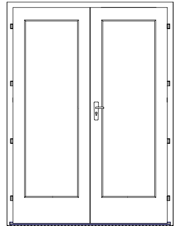
Double door 40 mm / 3mm 1425 x 1955 mm 1 st.
