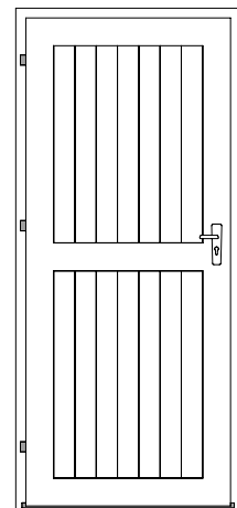
Door 40 mm 840 x 1835 mm 1 st.
