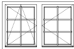
NR. 026 Doppelfenster ISO 70 mm 1530 x 990 mm 2 st.
