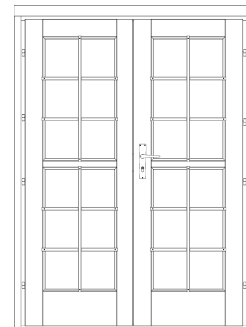
NR. 025 Doppeltür ISO 70 mm 1425 x 1955 mm 1 st.
